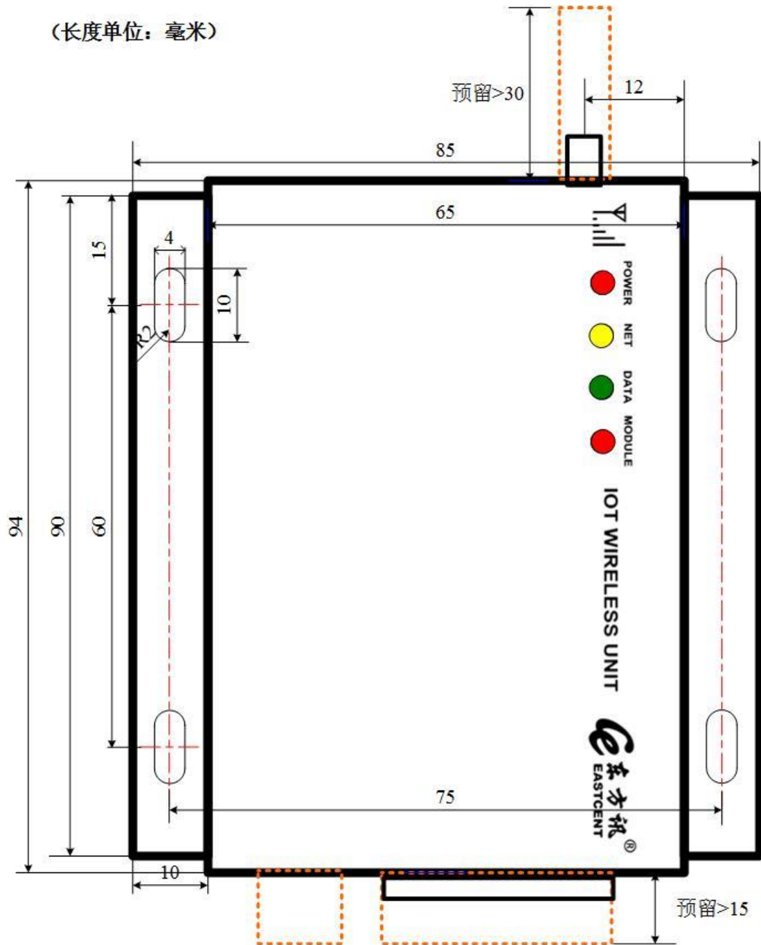
(图3) 产品外形尺寸图
